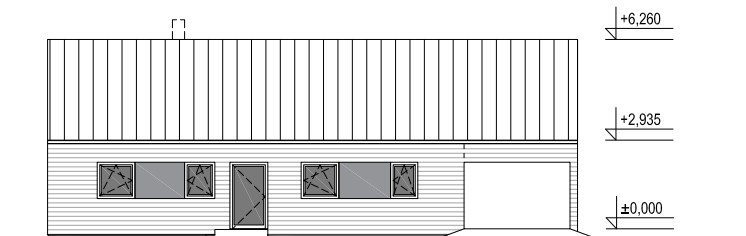
POHLED 1 M 1:250
