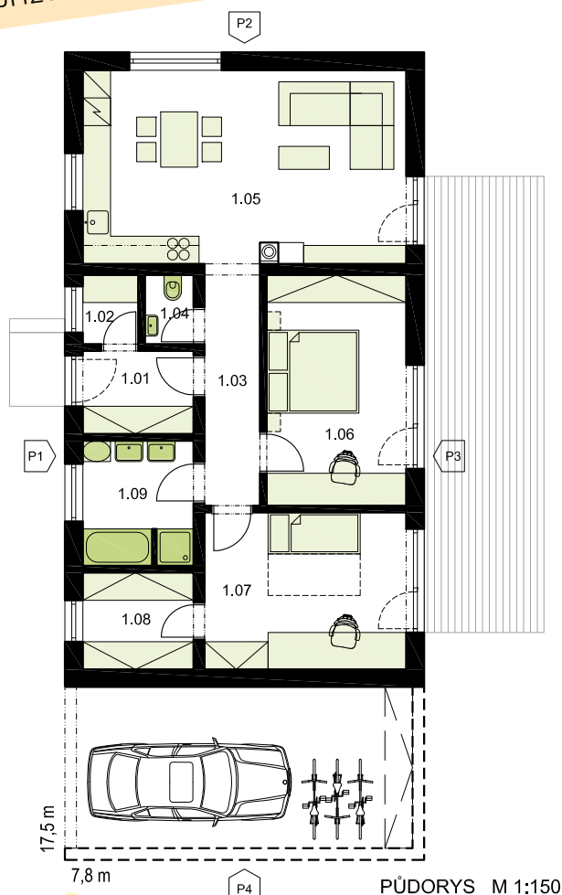
PŮDORYS M 1:150
