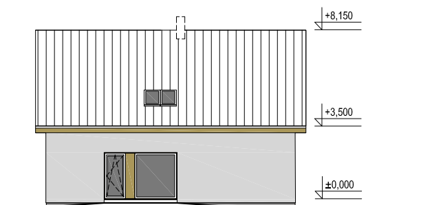
POHLED 3 M 1:250
