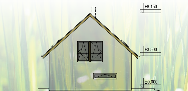
POHLED 4 M 1:250
