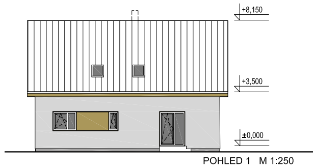
POHLED 1 M 1:250
