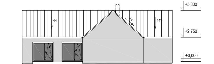
POHLED 1 M 1:250
