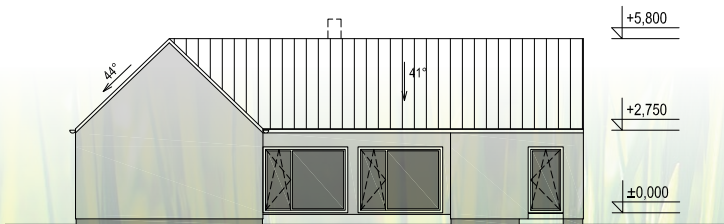
POHLED 4 M 1:250
