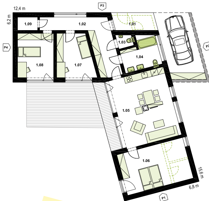
PŮDORYS M 1:200
