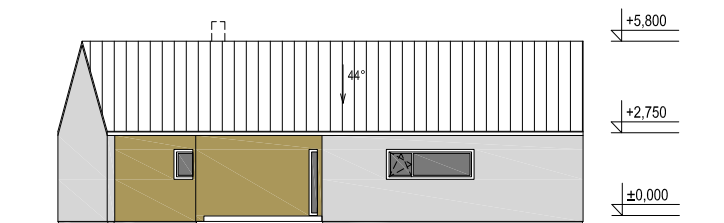
POHLED 3 M 1:250
