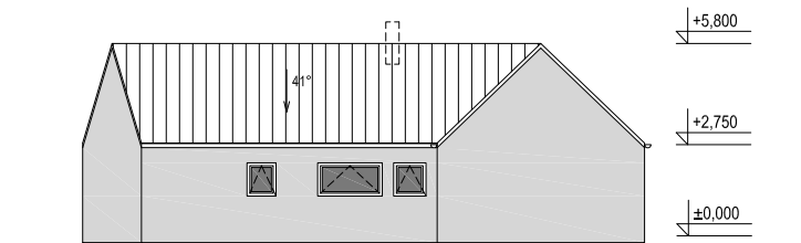
POHLED 2 M 1:250
